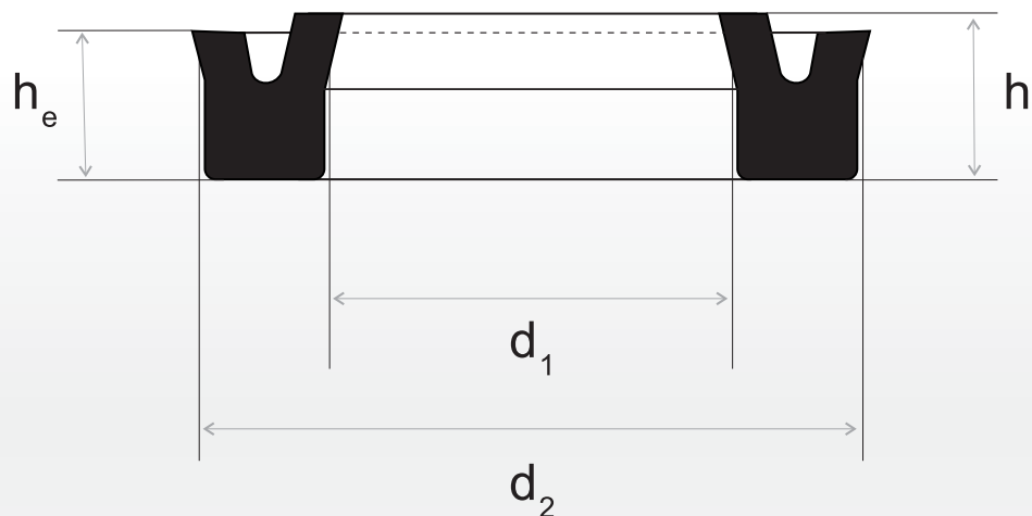
Seção típica de Gaxeta tipo "U"
