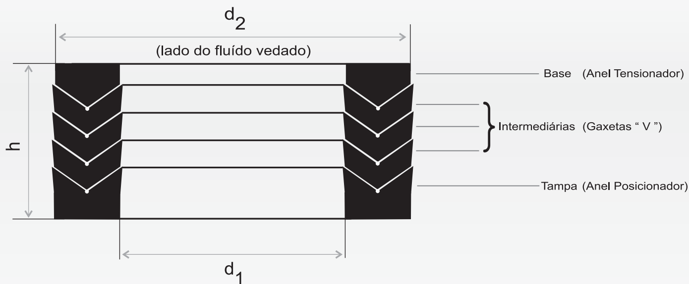
Seção de jogo de Gaxetas tipo “Chevron”
